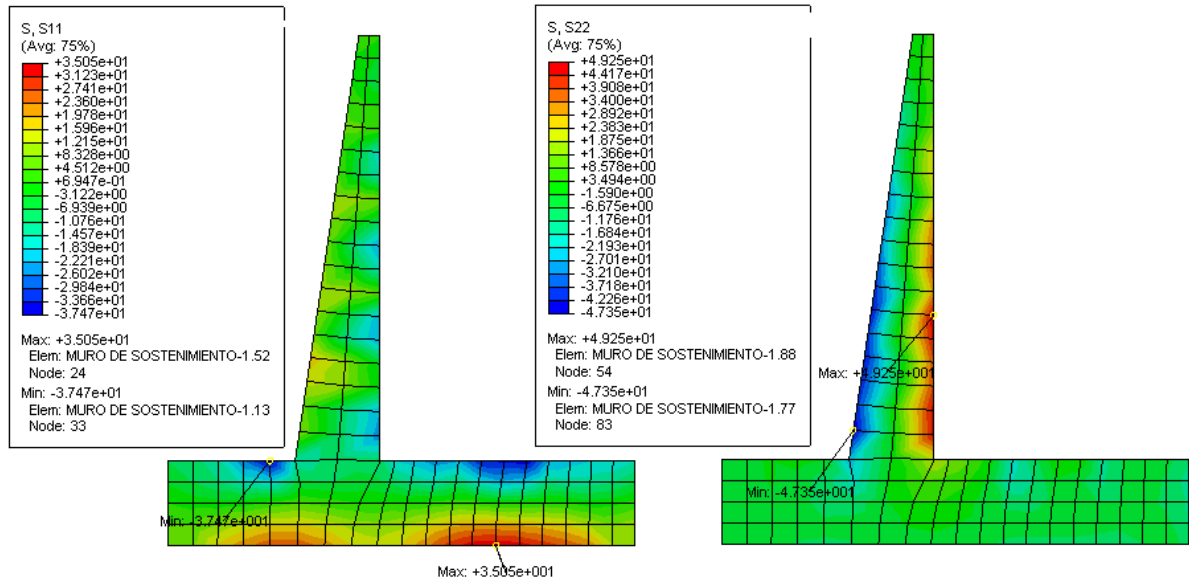
Figura 5.10: Tensiones S_{11} (Izquierda) y S_{22} (Derecha)
